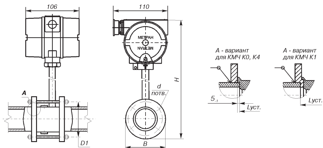
Рис. 10. Расходомер Метран-300ПР-А (Dy25...100); с подключением через штепсельный разъем (код "ШР").
