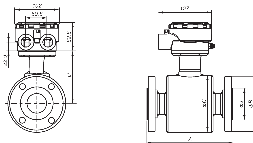
Рис. 4. Расходомер Rosemount 8750 Dy 15-100 мм (размеры см. табл. 6).
