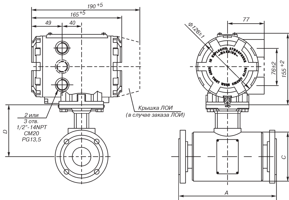
Рис. 5. Расходомер Rosemount 8700 с датчиком расхода 8705 или 8707 и преобразователем 8732Е (размеры см. табл. 9).
