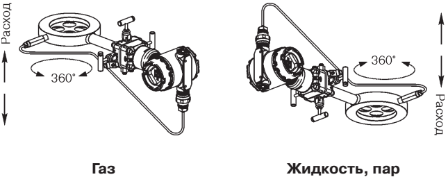
Рис.4. Допускаемые варианты установки расходомера при вертикальной ориентации трубопровода.
