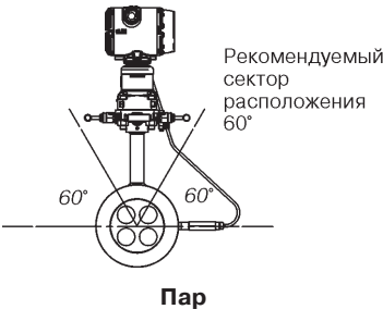
Рис.5. Монтаж сверху.
