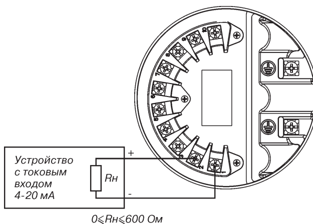
Рис.2. Схема подключения преобразователя 8732Е к контуру 4-20 мА.
