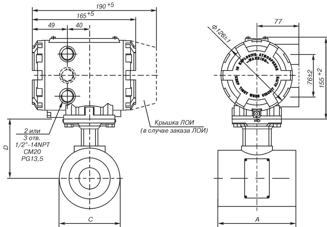
Рис.7. Расходомер Rosemount 8700 с датчиком расхода 8711 (Ду от 40 до 200) и преобразователем 8732Е (размеры см.табл.11).
