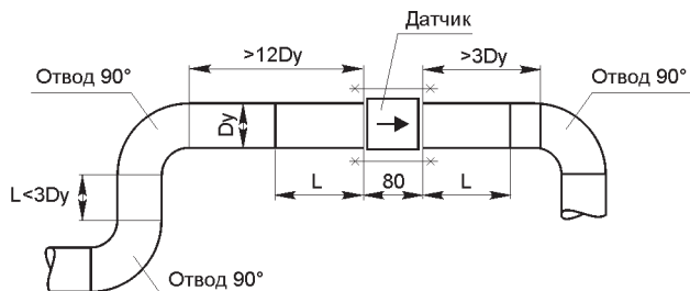
Рис.5. Установка в газопровод (паропровод) с отводом 90°.
