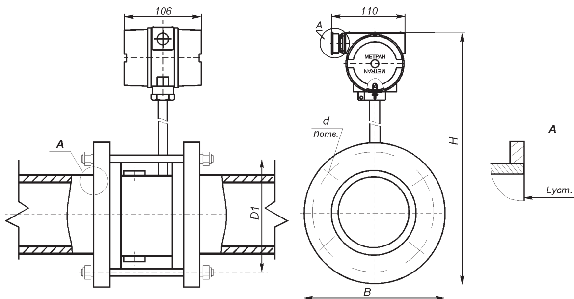
Рис. 11. Расходомер Метран-300ПР, Dy 250, 300; с подключением через штепсельный разъем (код "ШР").
