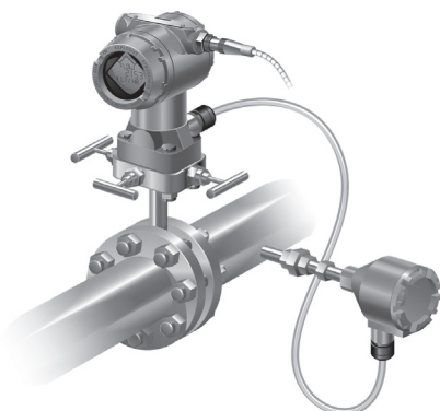
Рис. 1. Установка расходомера Rosemount 3051SMV.
