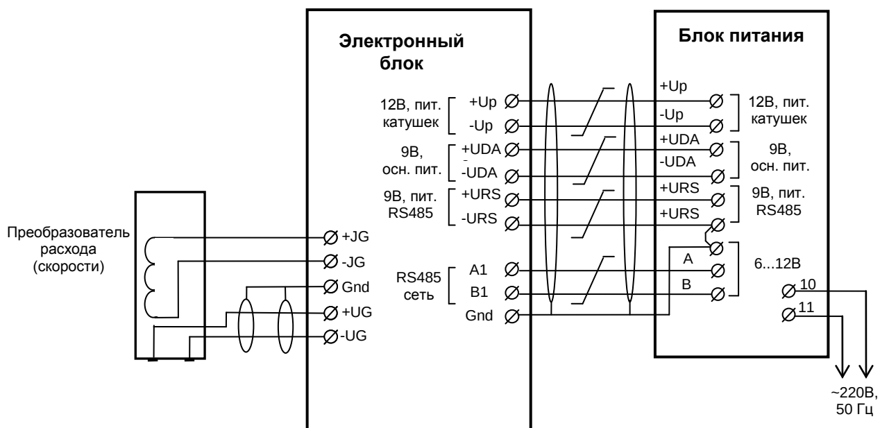
Рисунок А2 — Схема подключения при поверке преобразователей расхода (скорости)
