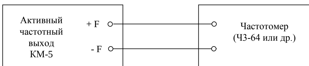
Рисунок А.6 — Схема подключения эталонного частотомера при поверке стандартных частотных выходов каналов КМ-5.
