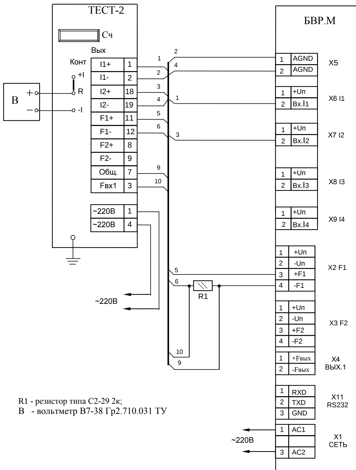
Рисунок К.1 – Схема проверки блока БВР.М
