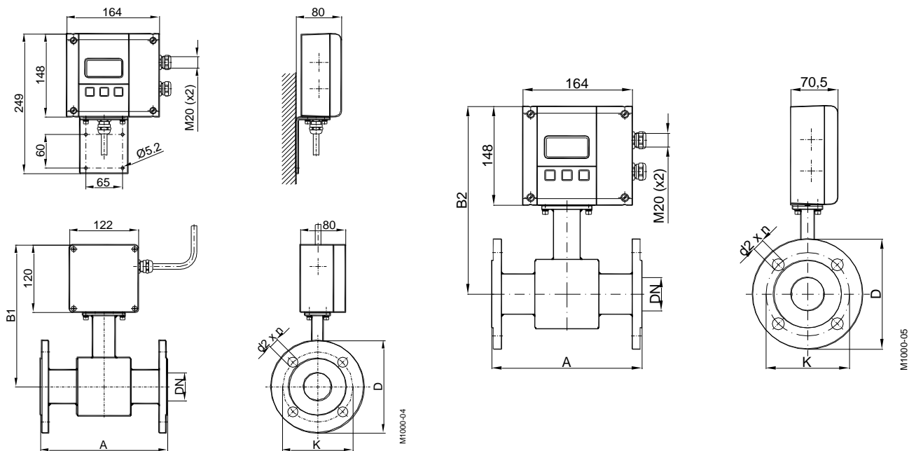
Фланцевое соединение ModMAG® M1000 раздельное исполнение
