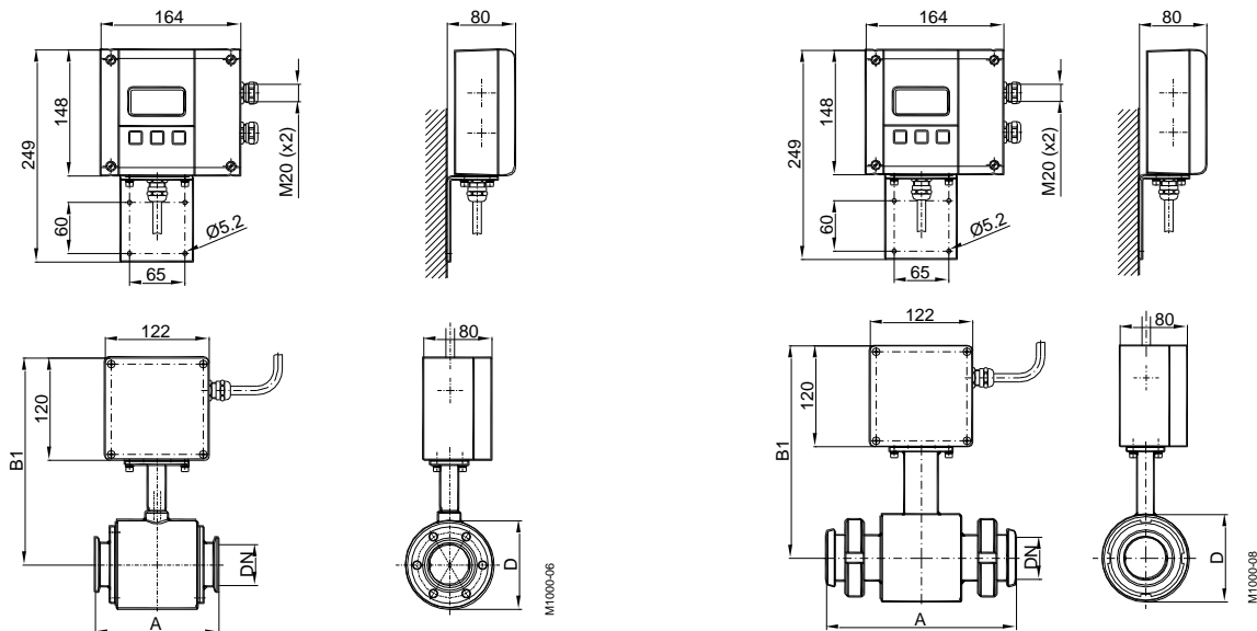
Соединение Tri-Clamp® ModMAG® M1000 раздельное исполнение
