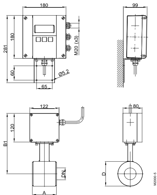
Sandwich connection M2000® отделенное исполнение
