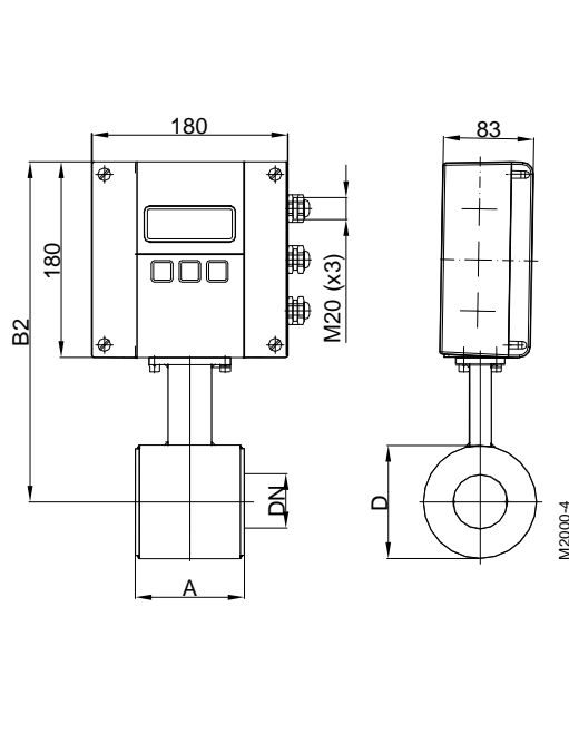
Sandwich connection M2000® компактное исполнение
