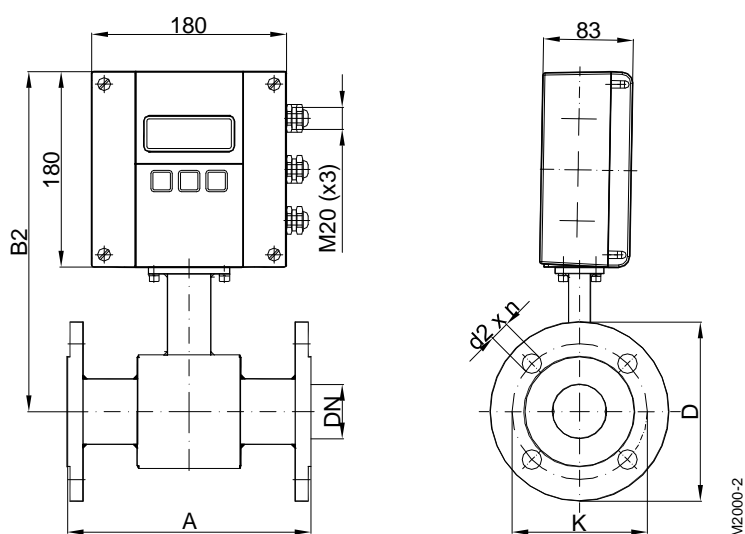
Process connection flange M2000® компактное исполнение
