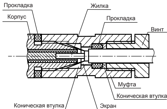
Рисунок 11 - Схема присоединения кабеля с ПЭП
