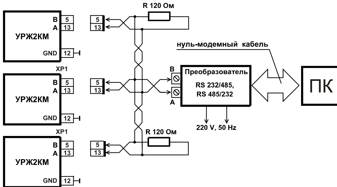
Рисунок E1 Схема локальной сети, выполненной посредством интерфейса RS 485 расходомера УРЖ2КМ Модель 1
