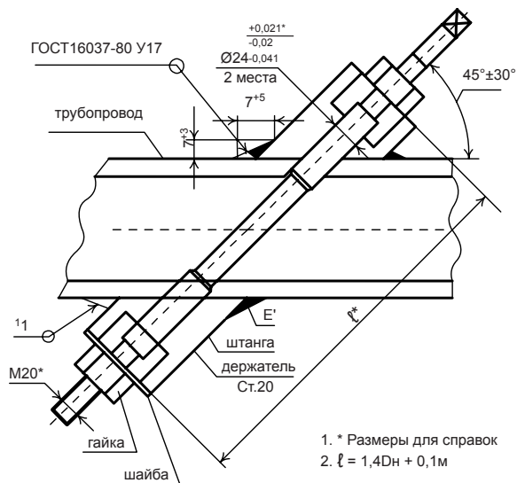
Рисунок 4 - Схема приварки держателей к трубопроводу
