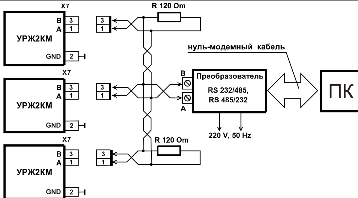
Рисунок Е2 Схема локальной сети, выполненной посредством интерфейса RS 485 расходомера УРЖ2КМ Модель 2
