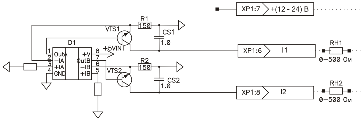
Рисунок Д1 Схема выходного каскада нормированного токового выхода расходомера УРЖ2КМ Модель 1
