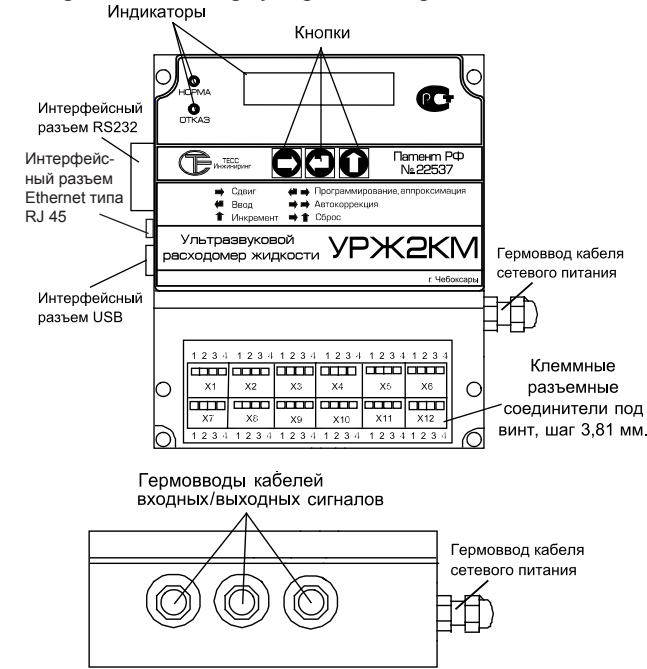
Рисунок 2. Расположение элементов управления, индикации и разъемов на корпусе расходомера УРЖ2КМ Модель 1
