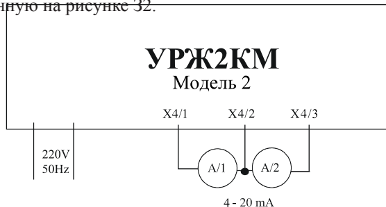
Рисунок 32. А/1, А/2 – ампервольтметр универсальный GDM-8245 или с не худшими характеристиками.
