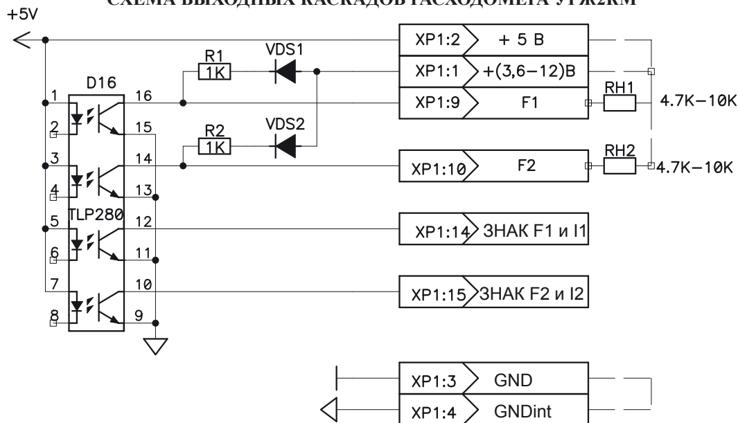
Рисунок Г1 Схема выходного каскада импульсного выхода и компаратора расходомера УРЖ2КМ Модель 1
