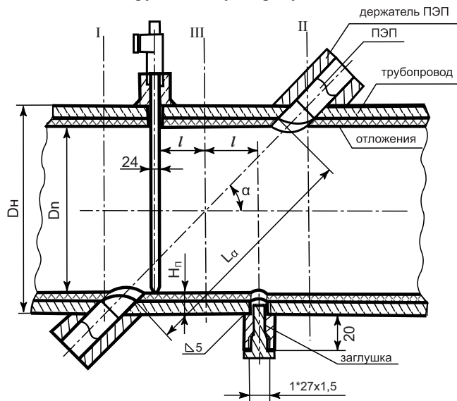
Рисунок 5 - Схема измерения суммарной толщины стенки трубопровода и отложений ( H_n )
