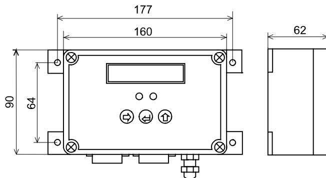
Габаритные размеры расходомера УРЖ2КМ Модель 1
