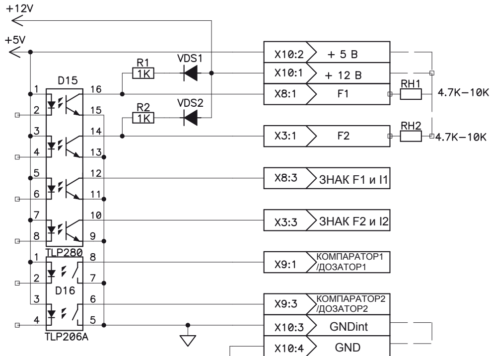
Рисунок Г2 Схема выходного каскада импульсного выхода и компаратора расходомера УРЖ2КМ Модель 2
