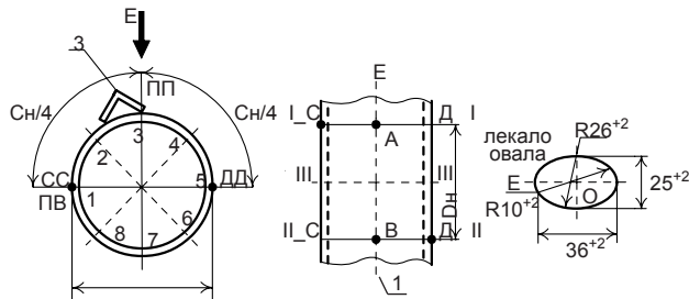
Рисунок 3 - Разметка трубопровода для приварки держателей ПЭП
