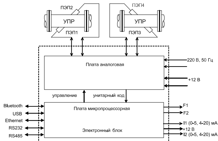
Рисунок 5. Структурная схема расходомера УРЖ2КМ Модель 2.
