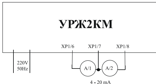
Рисунок 31. А/1, А/2 – ампервольтметр универсальный GDM-8245 или с не худшими характеристиками.
