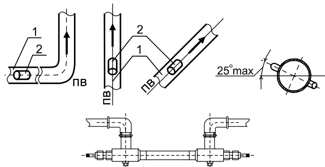
Рисунок 1 – Пример рекомендуемого расположения участка монтажа.
