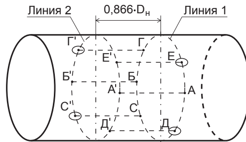
Рисунок 8 - Разметка трубопровода при врезке по хорде, вид с боку.
