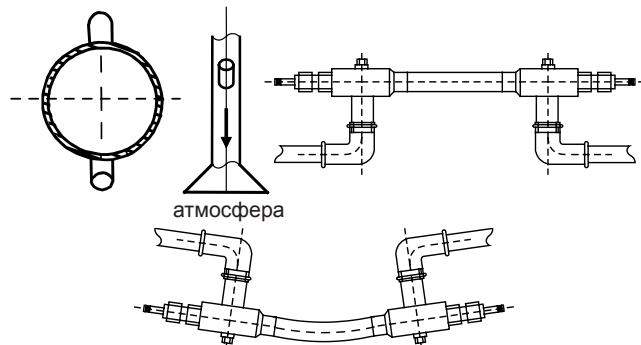
Рисунок 1 - Пример неправильного расположения измерительного участка
