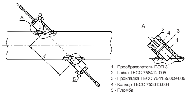
Рисунок 7 - Схема монтажа пьезопреобразователей
