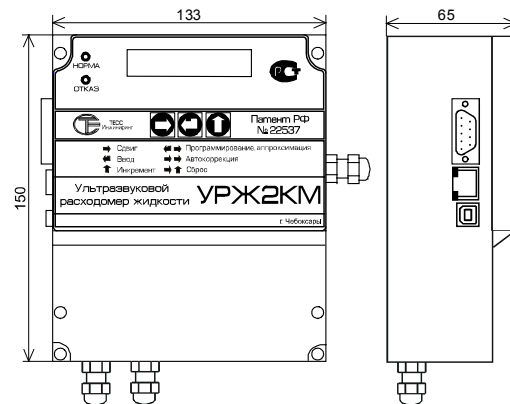
Габаритные размеры расходомера УРЖ2КМ Модель 2
