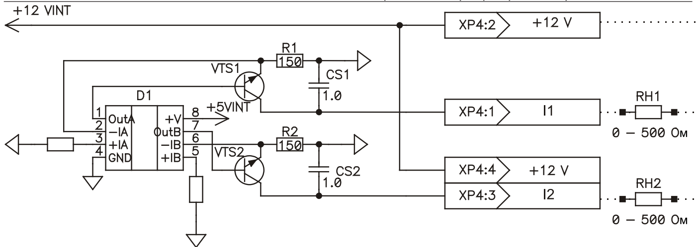
Рисунок Д2 Схема выходного каскада нормированного токового выхода расходомера УРЖ2КМ Модель 2
