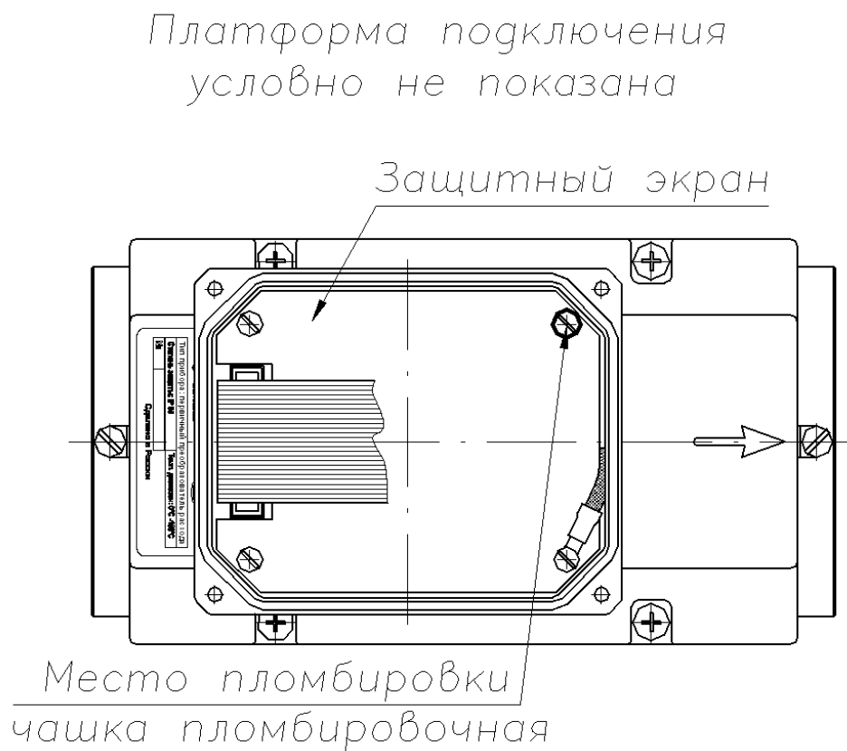
Рисунок Р.2 — Схема внутреннего пломбирования корпуса.
