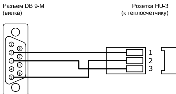
Рис. 9.5 Переходной кабель RS-232C (ТЭМ-104 - АПД)
