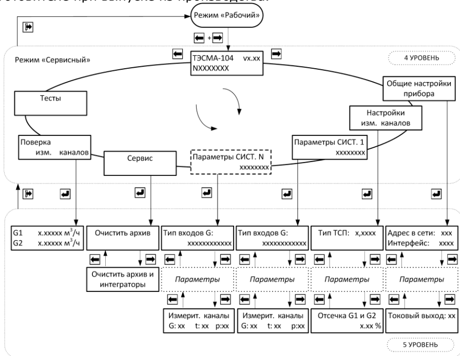
Рис. 9.3 Режим «Сервисный»
