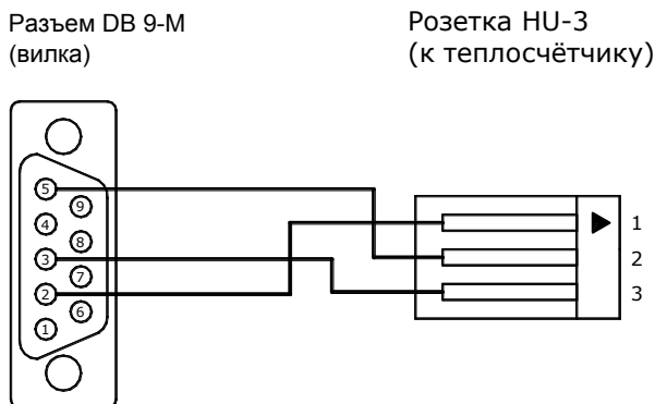
Рис. 7.4 Переходной кабель RS-232С (ТЭМ-106 – АПД)
