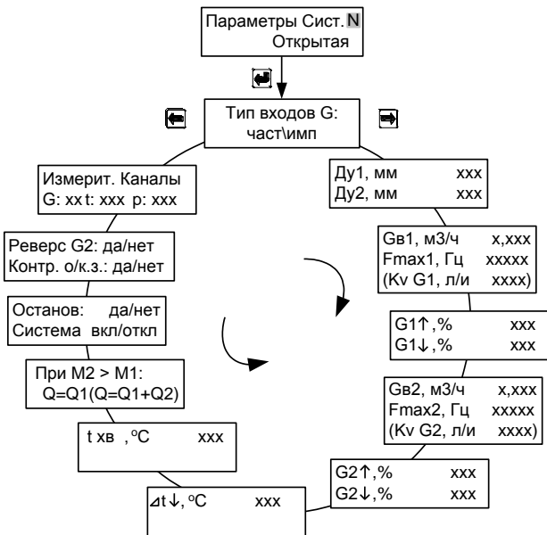
Рис. Д.6 Для теплосчётчика ТЭМ-106-01
