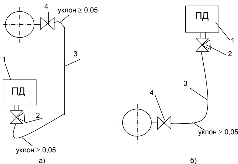
Рисунок 12 — Схемы присоединения датчиков давления на измерительном участке а) – датчик ниже отбора давления при измерении давления жидкости; б) – датчик выше отбора давления при измерении давления жидкости.
