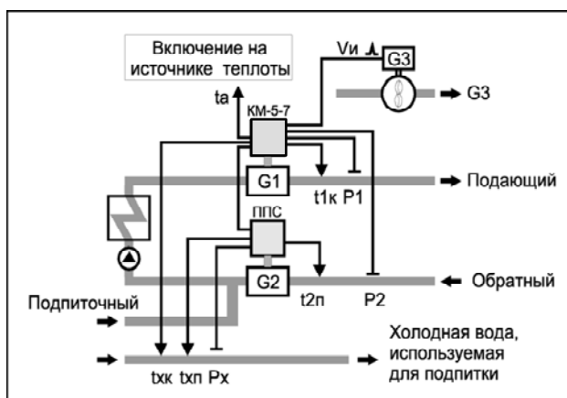
Алгоритм вычисления тепловой энергии теплосчётчика КМ-5-7
