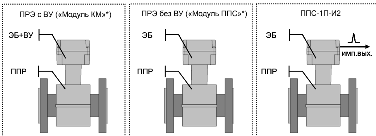
Рисунок 1а — Исполнение 1 ПРЭ и ППС-1П-И2 (моноблочное)
