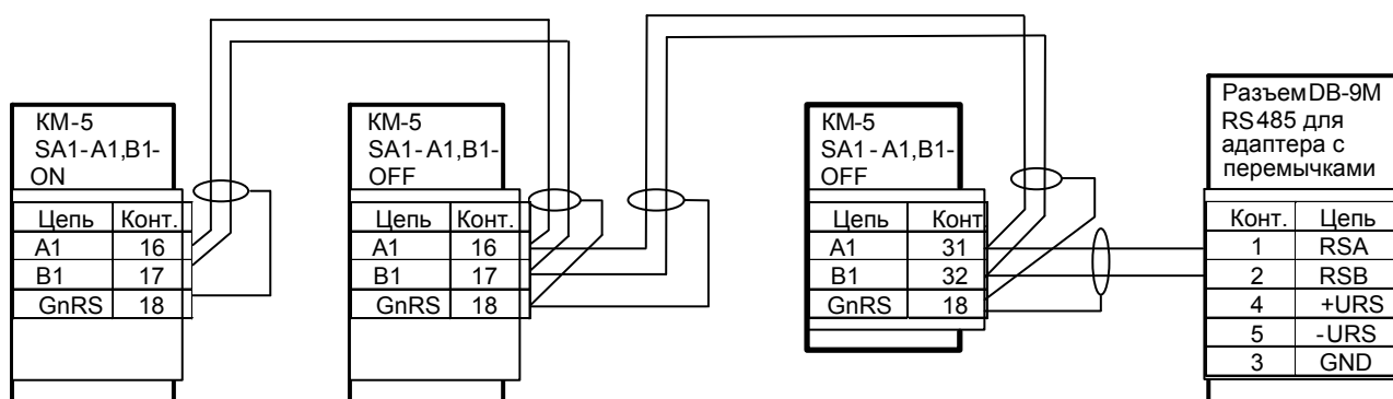
Рисунок Д.3 — Типовая схема сетевого соединения КМ-5
