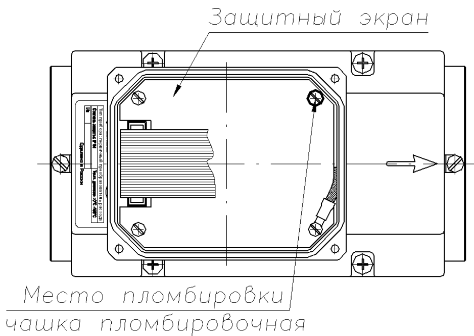
Рисунок В.3 — Схема внутреннего пломбирования корпуса
