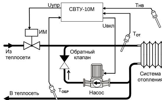
Рис.6 Регулирование температуры на выходе контура отопления с коррекцией по T_{нв} .
