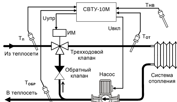
Рис.8 Регулирование температуры на входе контура отопления с коррекцией по Тнв и ограничением температуры "обратки".
