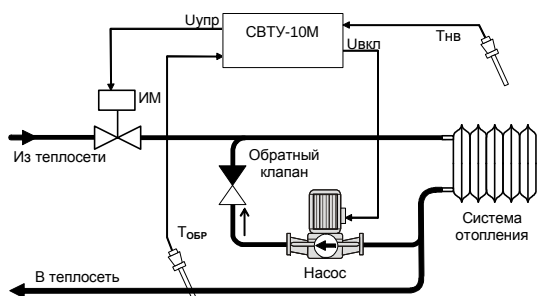
Рис.3 Регулирование температуры на выходе контура отопления с коррекцией по T_{нв}
