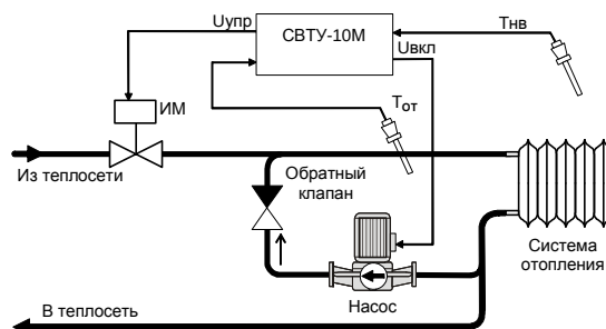
Рис.4 Регулирование температуры на входе контура отопления с коррекцией по T_{нв}
