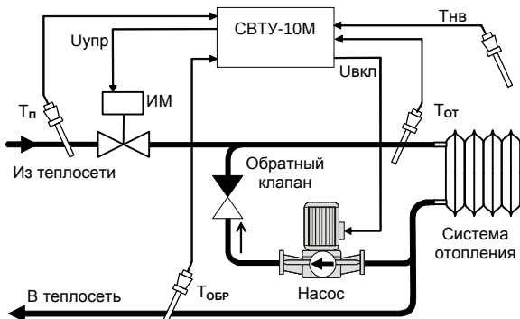
Рис.7 Регулирование температуры на входе контура отопления с коррекцией по Тнв и ограничением температуры "обратки".
