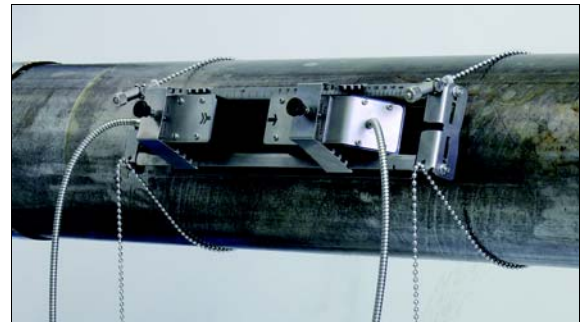
Измерение датчиками, смонтированными на портативном Variofix VP
